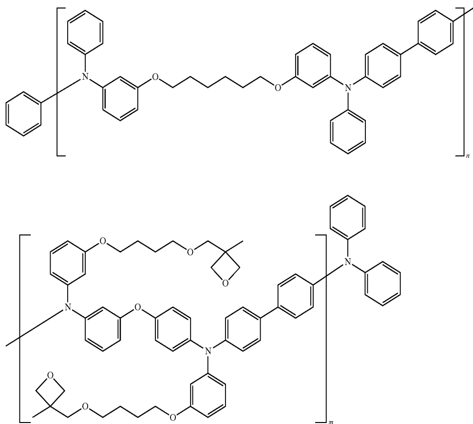
[Formula 35]
