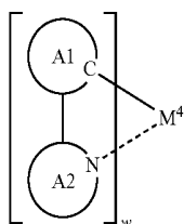
[Formula 59]
