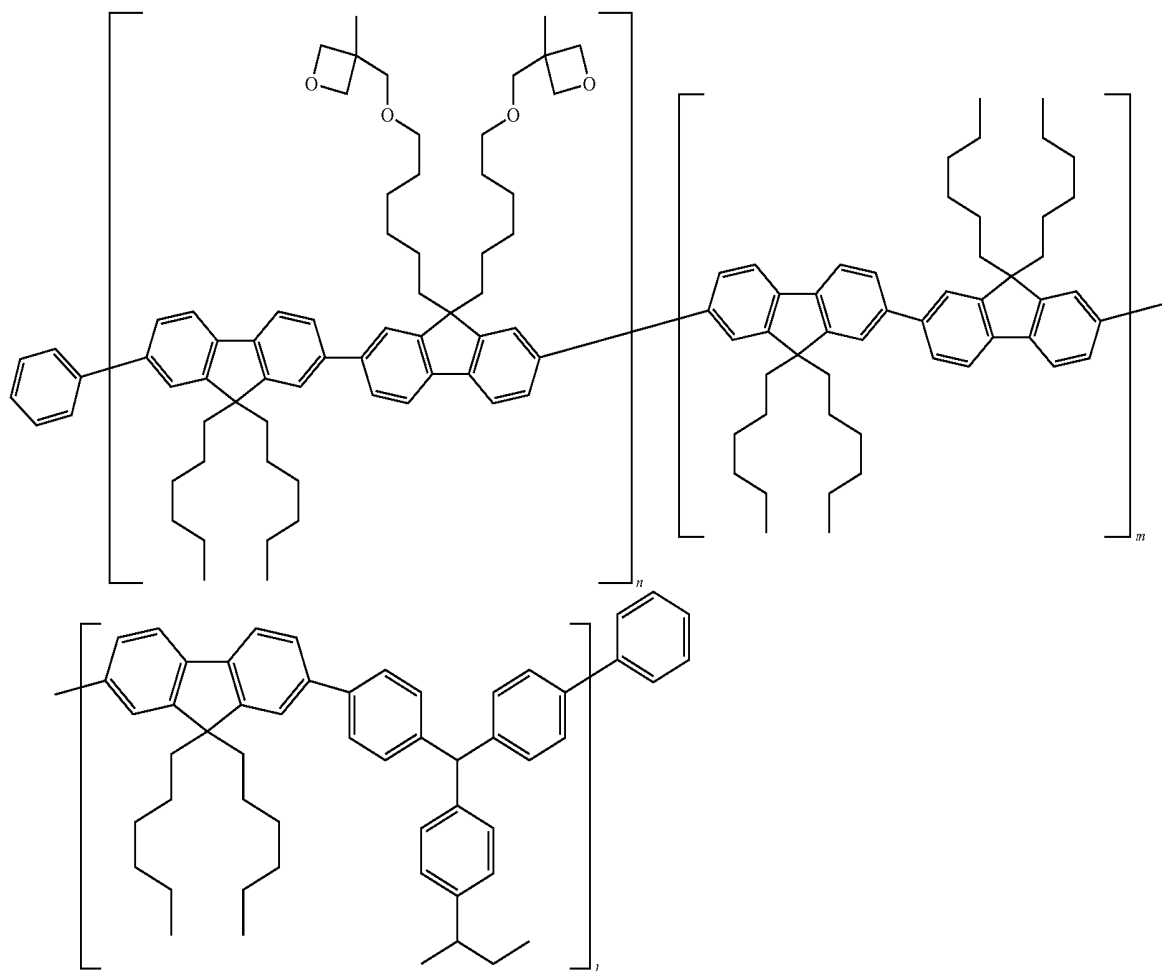
[Formula 38]
