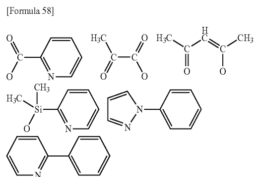
[Formula 58]
