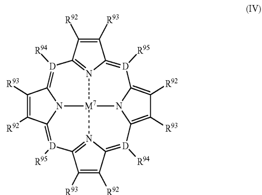
[Formula 55]
